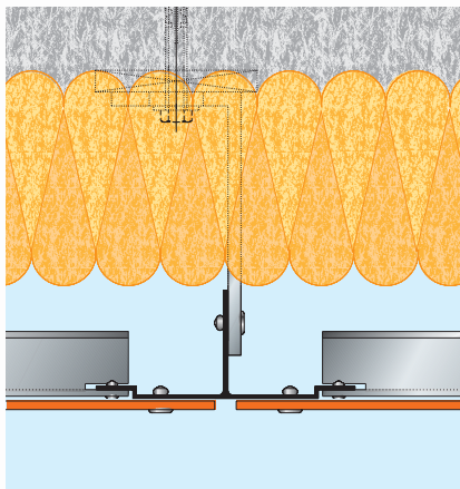
Horizontalschnitt
