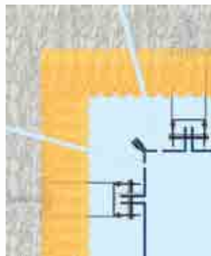
Fassaden-Innenecke - Horizontalschnitt
