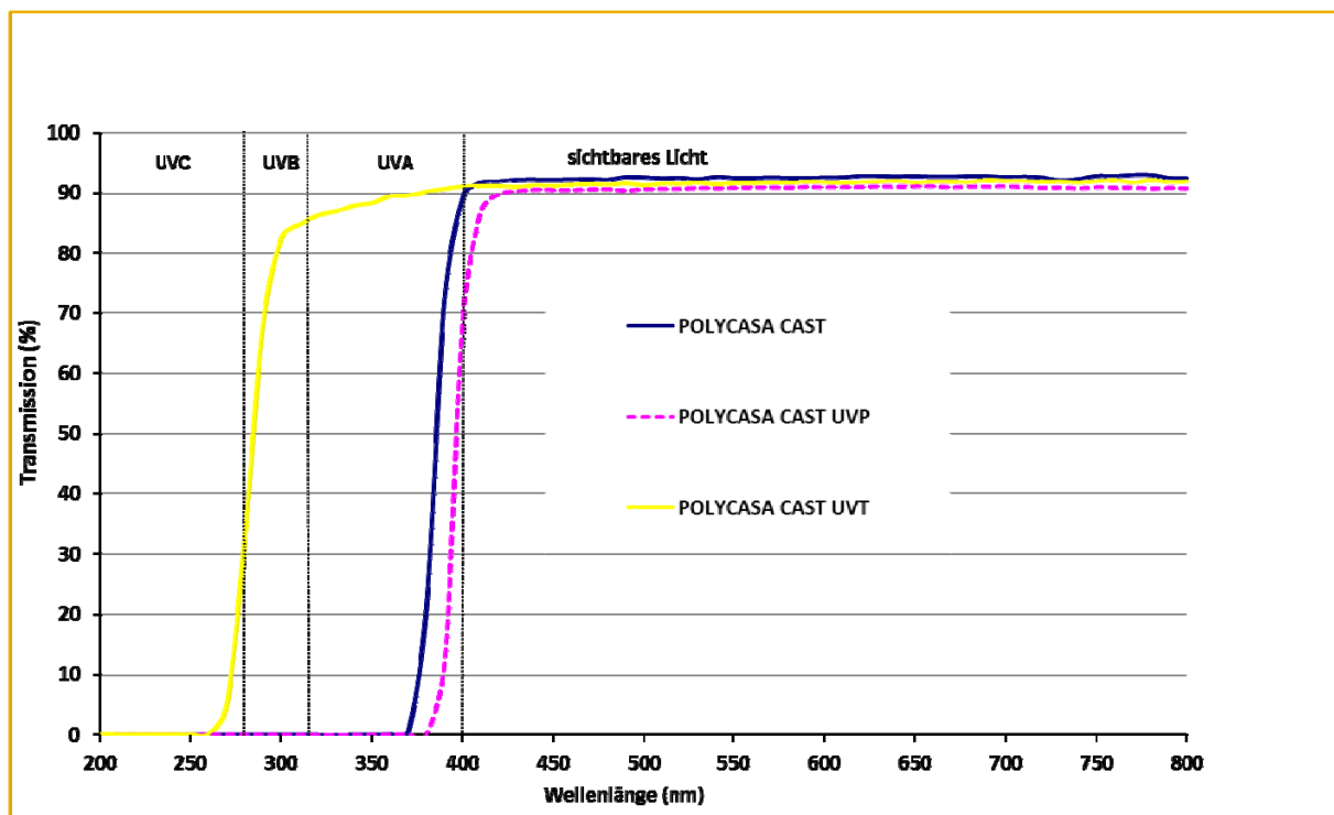
Transmissionsspektren von POLYCASA CAST Standard, UVP und UVT.
